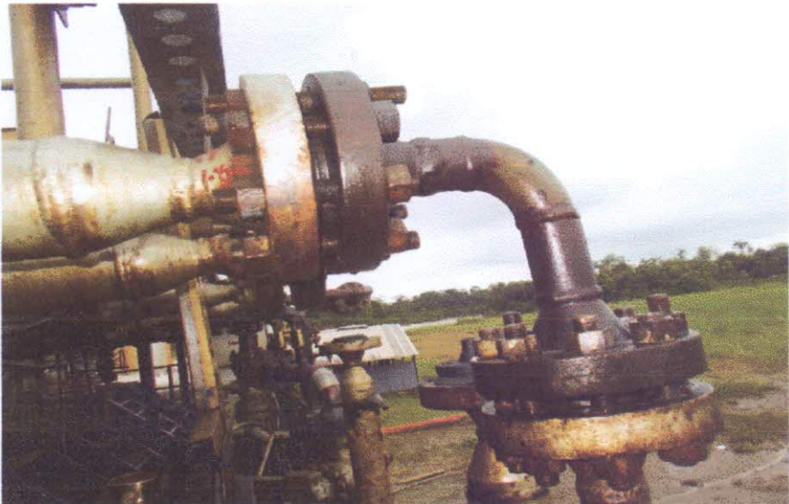
SPILL POINT ELBOW SHOWN: fig2
